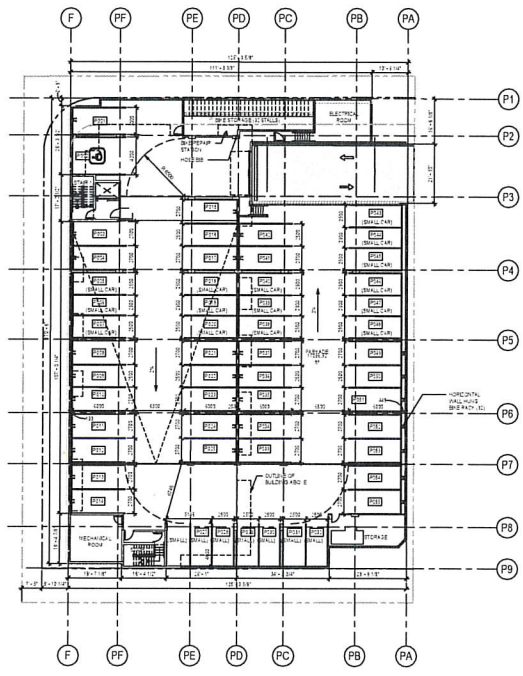
1 FLOOR PLAN - P1 SCALE: 1/8" = 1'-0"
